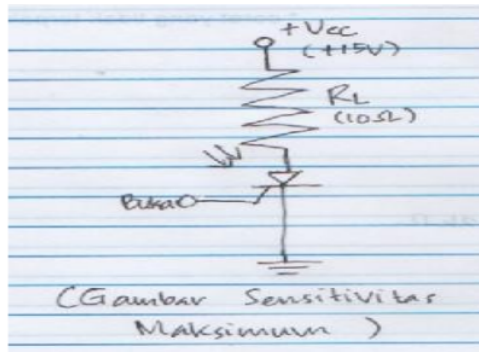
Gambar 4. Contoh jawaban mahasiswa pada soal tiristor ( LASCR )
