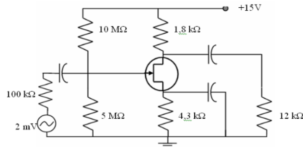
Gambar 1. Rangkaian penguat sumber sekutu
