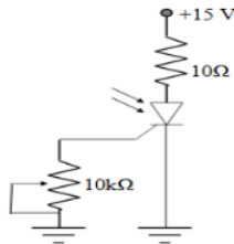
Gambar 3. sakelar penahan menggunakan LASCR
